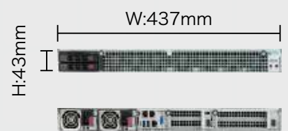
製品サイズ
