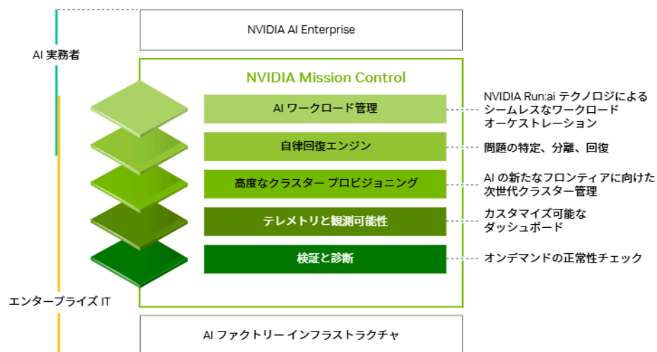
NVIDIA DGX ソフトウェアスタック
